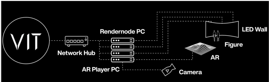
<그림 3> VIT의 장비 연결 구조
