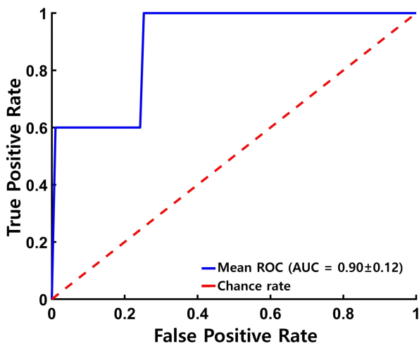
그림 9. 사용자 분류 모델의 평균 ROC 커브 Fig. 9. Average ROC of the user classification model
