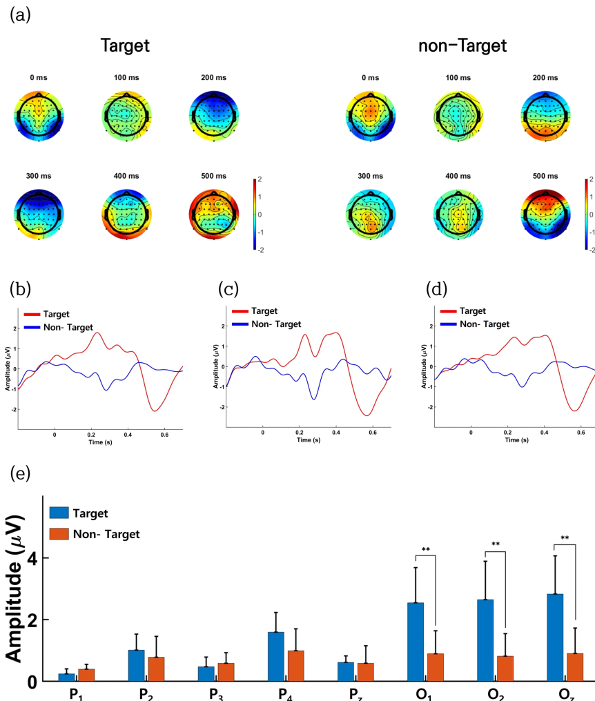
그림 5. (a) 알파벳 이미지 기반의 10 Hz grow/shrink 프로토콜 목표 자극(Target)과 표준 자극(Non-target)의 topographical maps. (b) O 1 , (c) O 2 , (d) O z 영역의 목표 자극과 표준 자극에 반응한 뇌파 시계열 데이터. (e) 5명의 실험참가자에 대한 목표 자극과 표준 자극의 P300 진폭 데이터(n=5, mean±1S.D) Fig. 5. (a) Topographical maps of 10 Hz growth/shrink protocol targets and non-target stimuli based on alphabetical images. (b) EEG time-series data of target and non-target stimuli at the (b) O 1 , (c) O 2 , and (d) O z area. (e) P300 amplitude data of target and non-target stimuli for 5 experimental participants (n=5, mean±1S.D)
