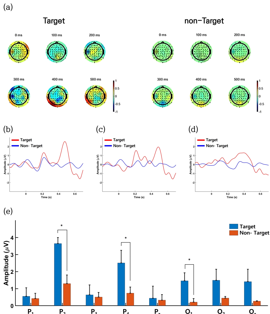
그림 3. (a) 조류 이미지 기반의 5 Hz flicker 프로토콜 타겟과 논-타겟 자극의 topographical maps. (b) P 2 , (c) P 4 , (d) O 1 영역의 목표 자극(Target)과 표준 자극(Non-target)의 뇌파 시계열 데이터. (e) 4명의 실험참가자에 대한 목표 자극과 표준 자극의 P300 진폭 데이터 (n=4, mean±1S.D)
