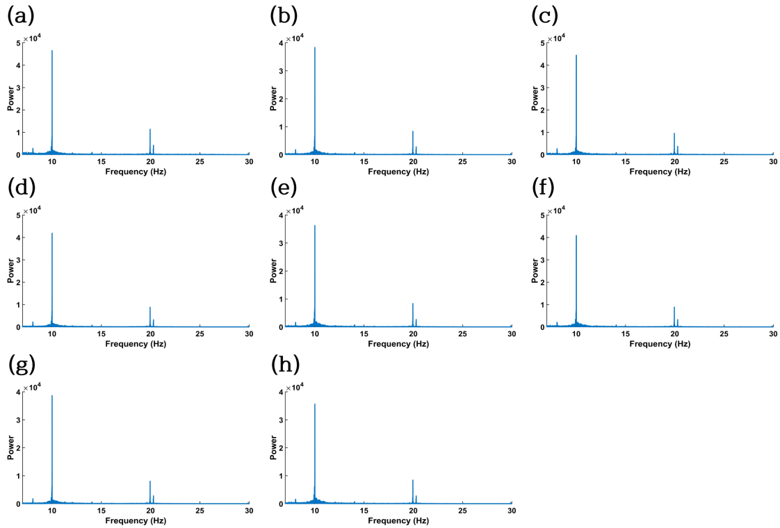
그림 6. (a) P 1 , (b) P 2 , (c) P 3 , (d) P 4 , (e) P z , (f) O 1 , (g) O 2 , (h) O z 영역에서의 10 Hz grow/shrink 시각 자극에 반응한 SSVEP 데이터의 power spectrum density
