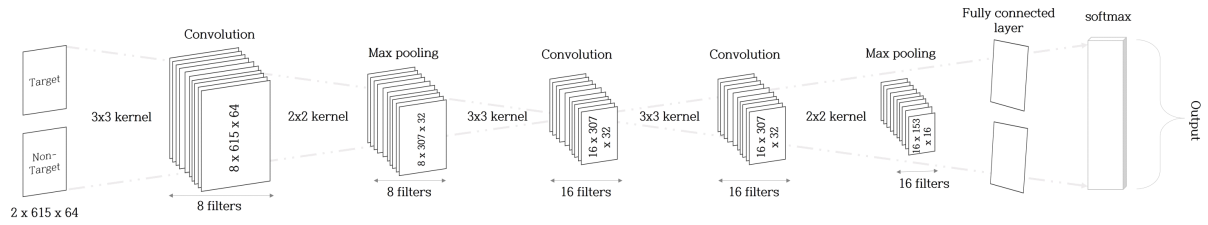
그림 7. 목표 자극(target)과 표준 자극(non-target) 분류를 위한 2D-CNN 아키텍처 Fig. 7. 2D-CNN architecture for target and non-target data classification
