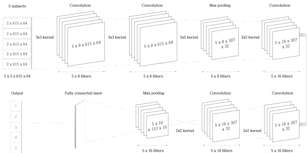
그림 8. 사용자 분류를 위한 2D-CNN 아키텍처 Fig. 8. 2D-CNN architecture for user classification
