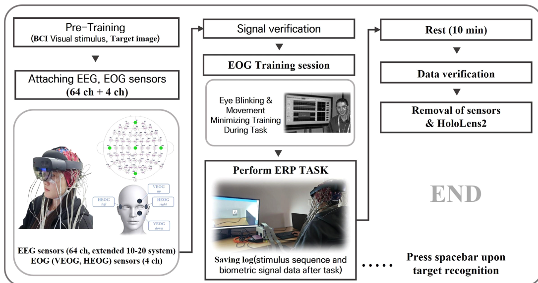
그림 2. SSVEP & P300 BCI 기반 사용자 인증 시스템 실험 절차
